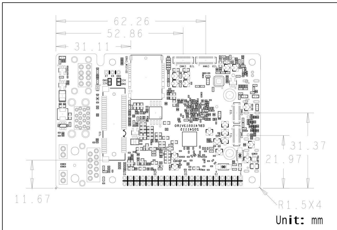
图 4.2-2 鲁班猫 3 背面机械尺寸图
